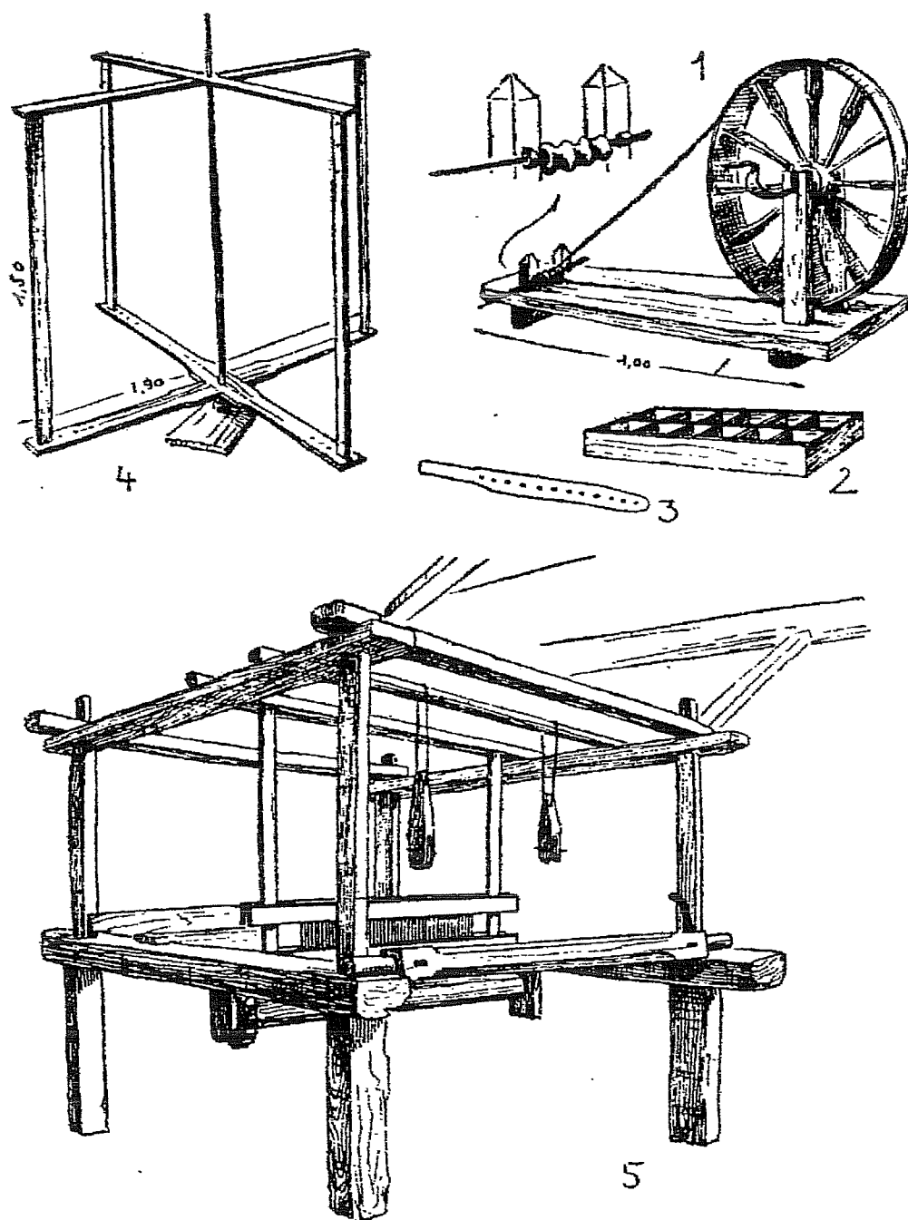
Fig. 39 — 1 Rodeleira; 2 Cassuleiru; 3 Escoiedeira; 4 Urdidor; 5 Telar.
