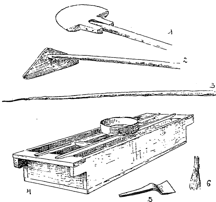
Fig. 18 — 1 Pala; 2 al rôdru; 3 Furgãeiro; 4 Maseira com bariêlas e peneira; 5 Raspadeira; 6 Bardeiro.
