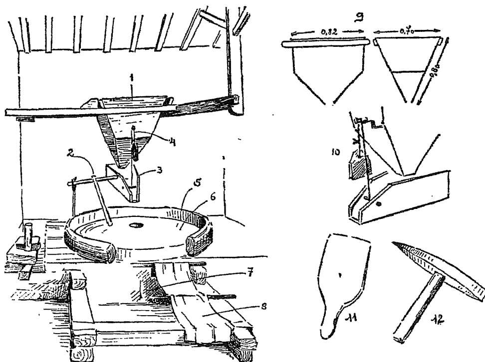
Fig. 19 — Moinho — 1 Tremoia; 2 Tarabêlo; 3 Caneleia; 4 Baraça; 5 Cambas ou cambões; 6 Piêdra de riba; 7 Farneiro; 8 Colador; 9 Tremoia de frente e de perfil; 10 Maneira de prender a baraça; 11 Pala dal farneiro; 12 Picas.
