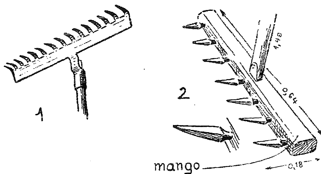
Fig. 31 — 1 Rastro de ferro; 2 Rastro de madeira.
