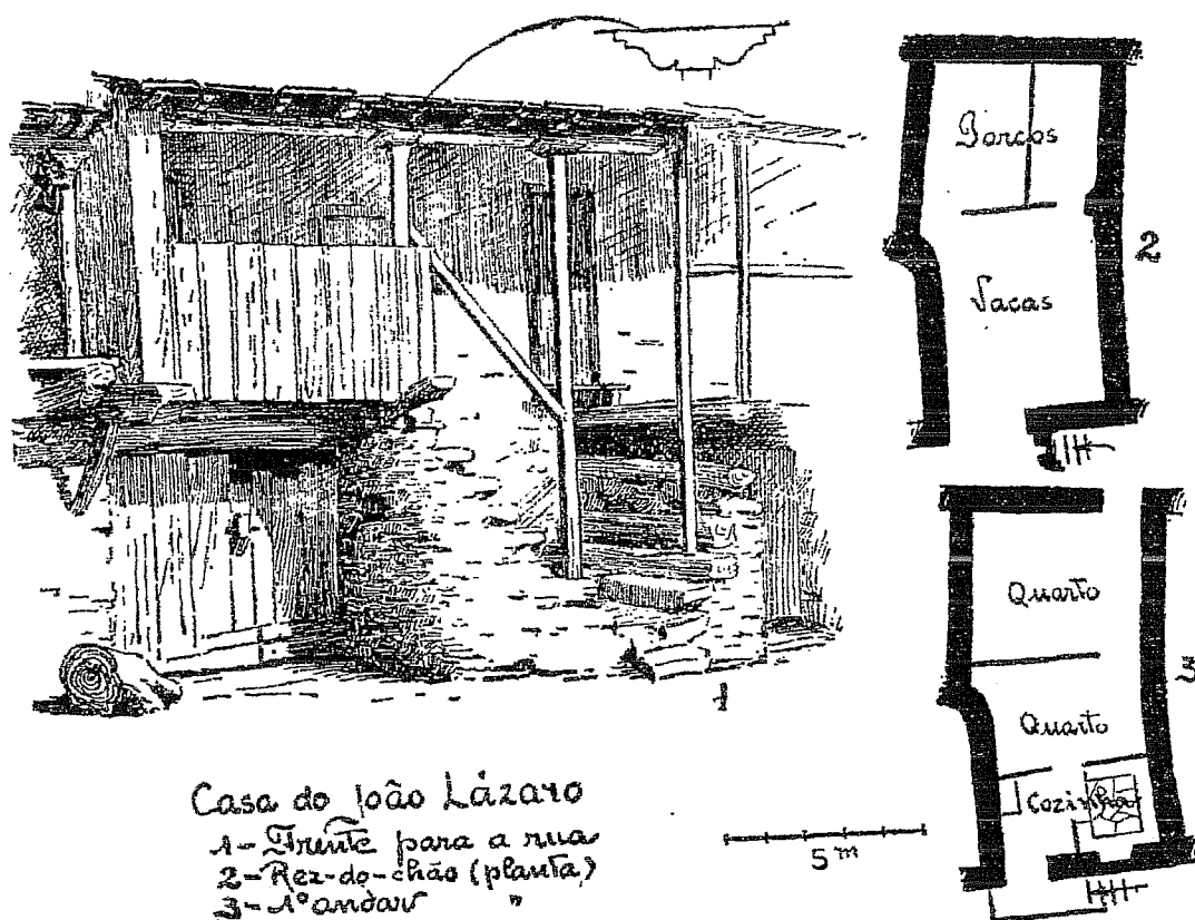
Fig. 7 — Casa do Tio Lázaro com a respectiva planta.
