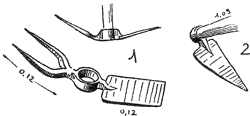
Fig. 26 — 1 Guintchas de rabo; 2 Satcho.
