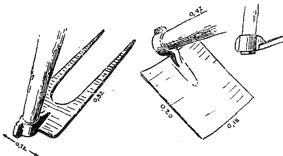
Fig. 25 — Gvintcha e sadantcha.
