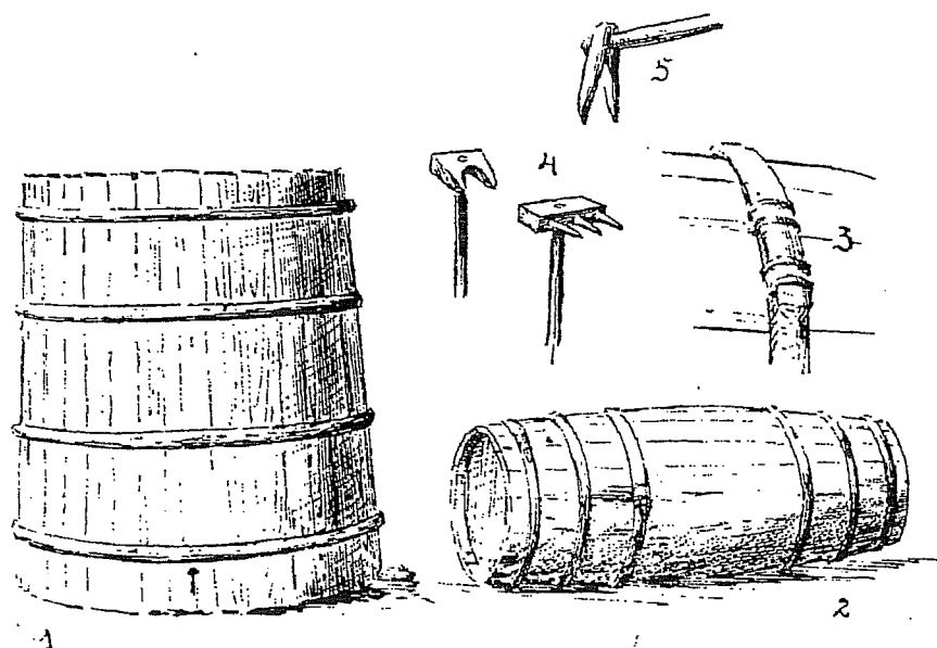
Fig. 21 — 1 Tina; 2 Pipa alongada comum na região; 3 Arco de madeira ainda usado em algumas tinas e pipas; 4 Ancinho de três dentes; 5 Ancinho bifurcado, usado para tirar o bagaço no alambique.
