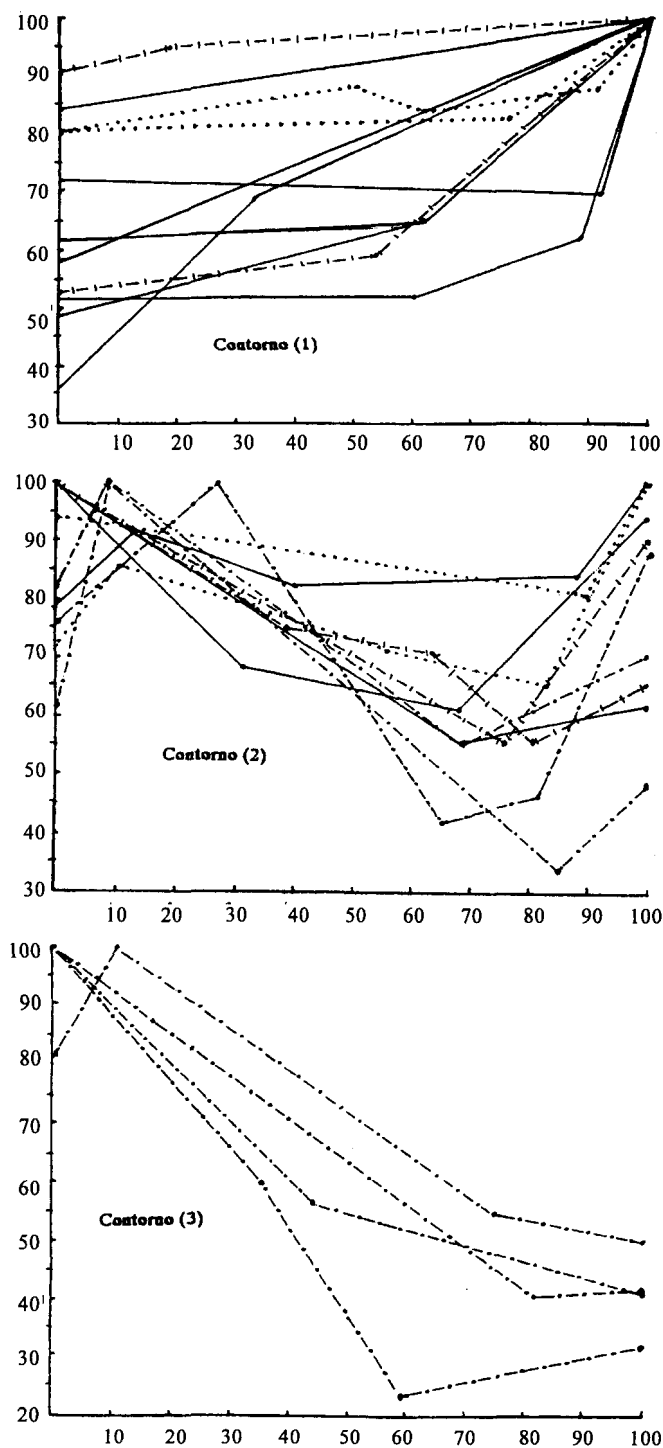
FIGURA 7 Interrogativa – Representação normalizada dos contornos entoacionais
