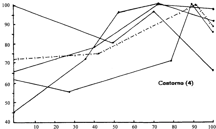
FIGURA 6 Declarativa – Representação normalizada dos contornos entoacionais
